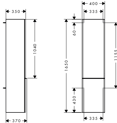
door hinge left
