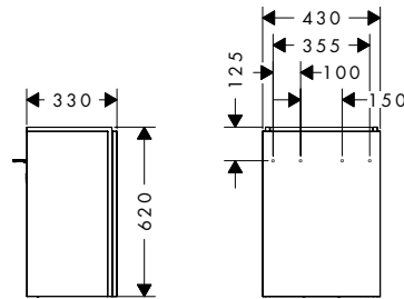
door hinge right
