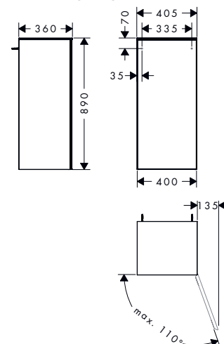
door hinge right
